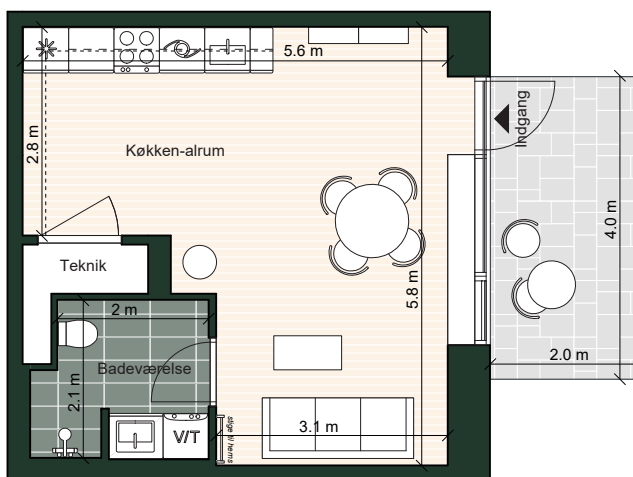
Stueplan
