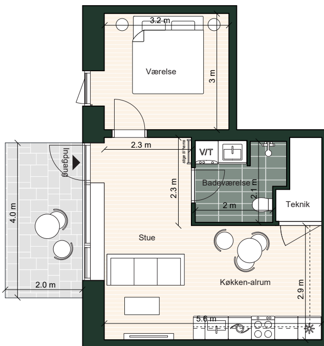
Stueplan
