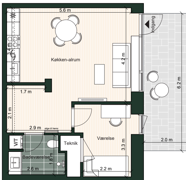
Stueplan
