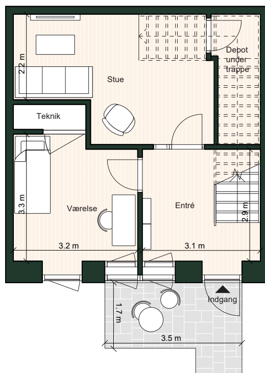
Stueplan
