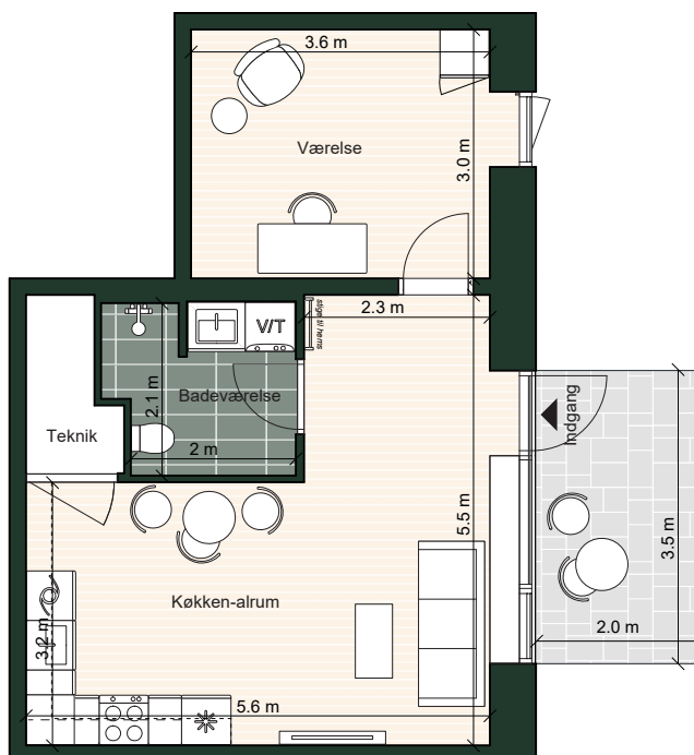
Stueplan
